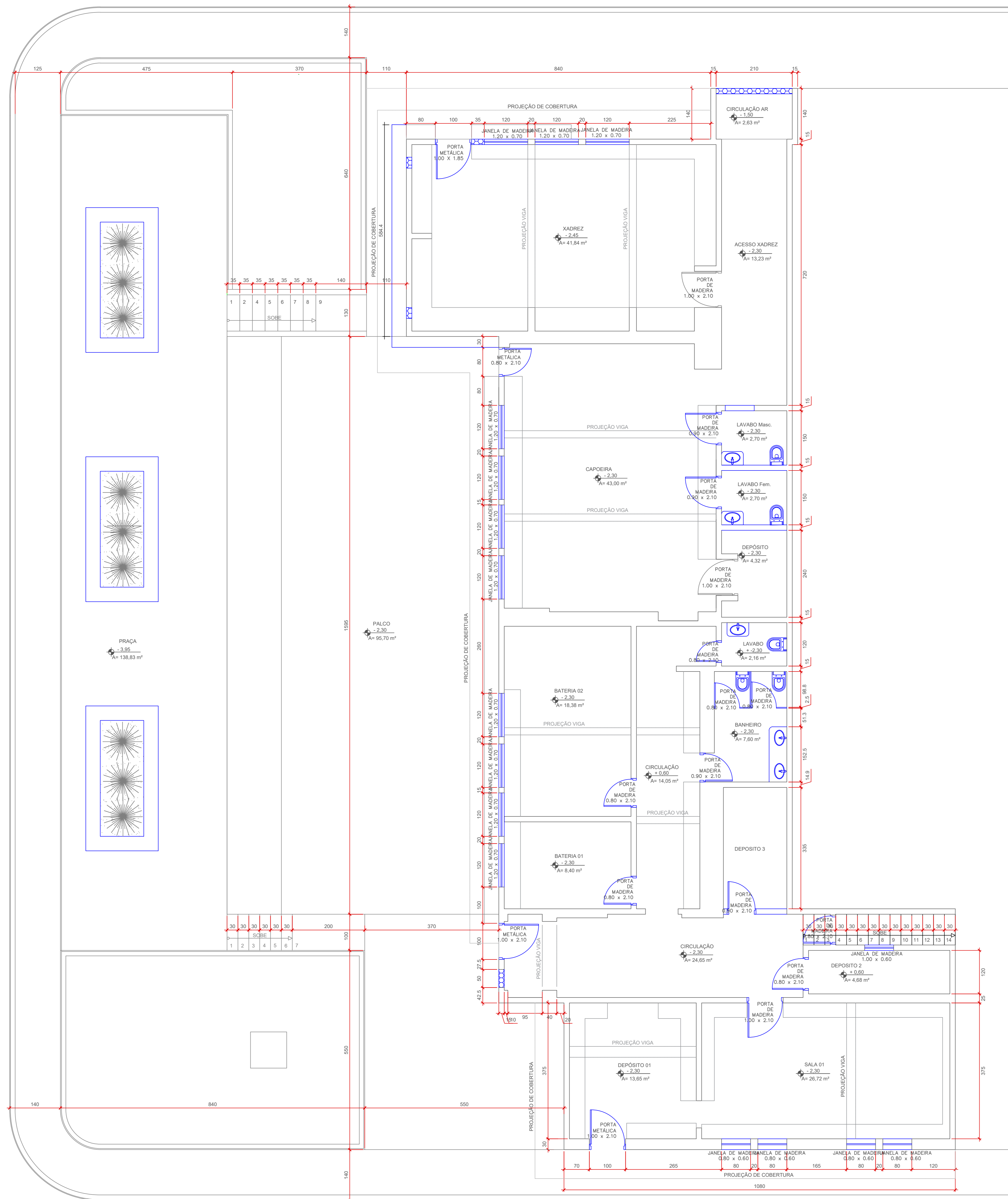
PLANTA BAIXA SUBSOLO N. -195 ESC.: 1:50
