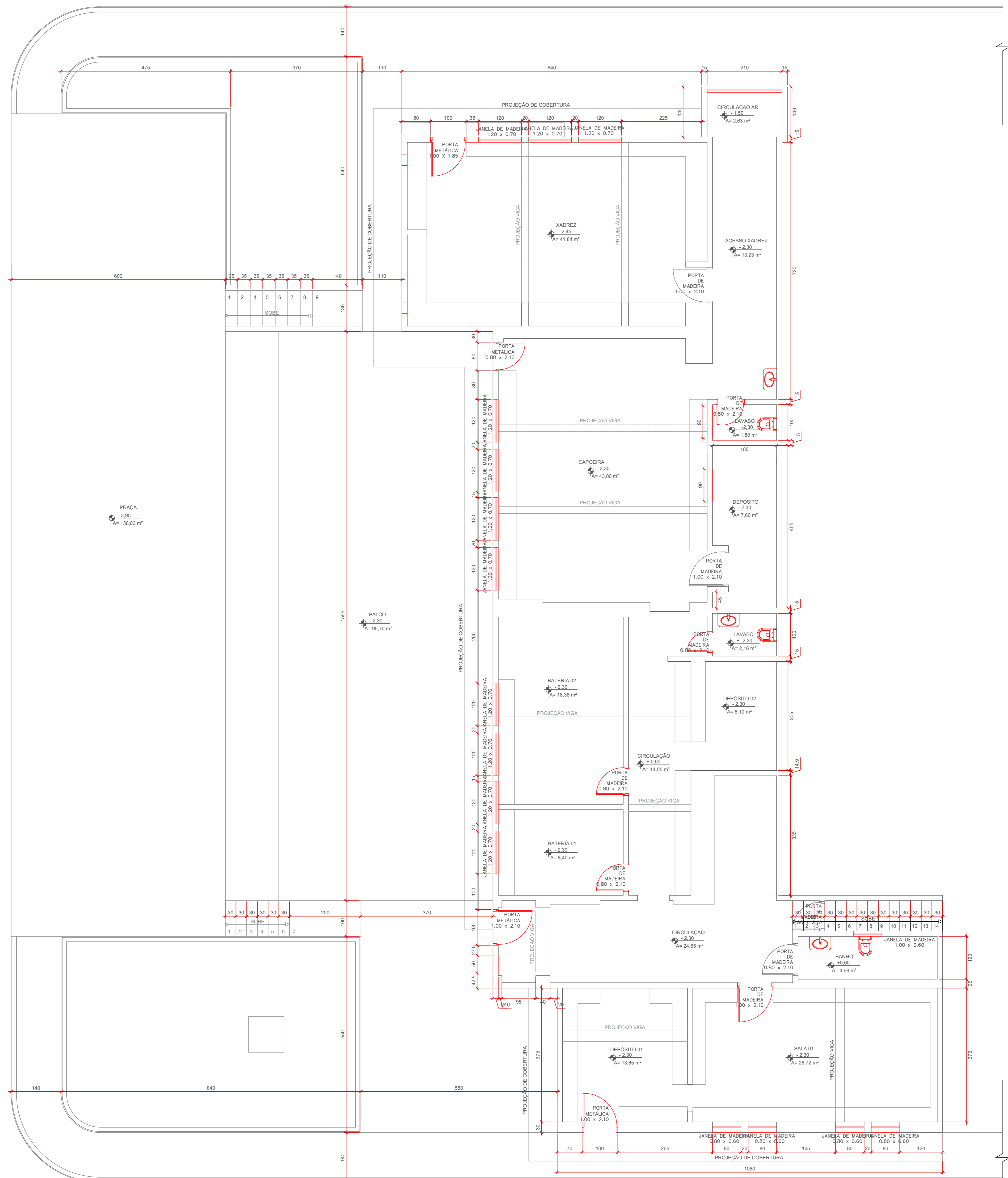
PLANTA DE DEMOLIÇÃO SUBSOLO ESC.: 1:50
