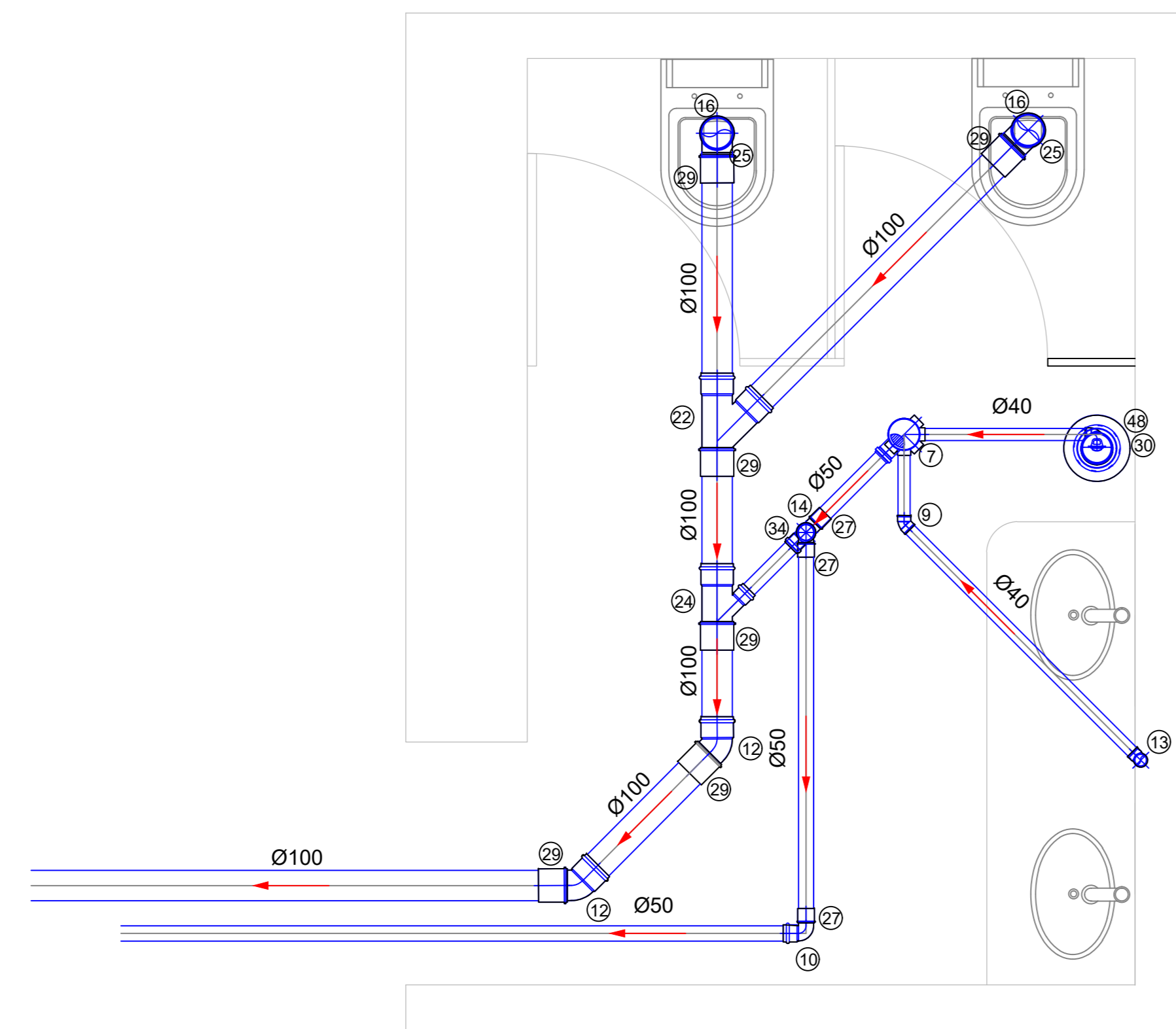
DETALHE 3 (1x) DETALHE DO BANHEIRO Escala 1:25
