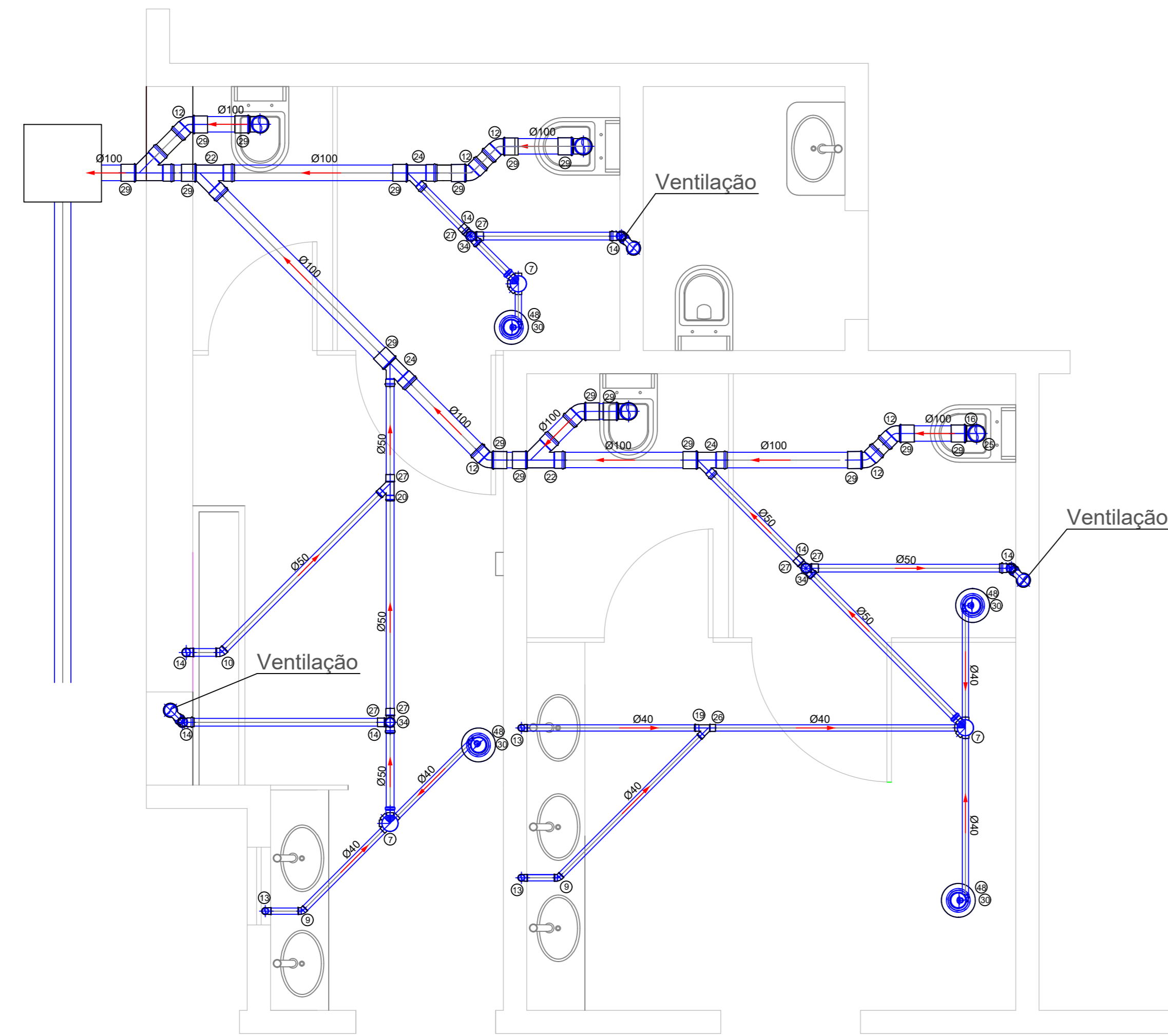
DETALHE 1 (1x) DETALHE DO BANHEIRO MASC. E FEM. Escala 1:25
