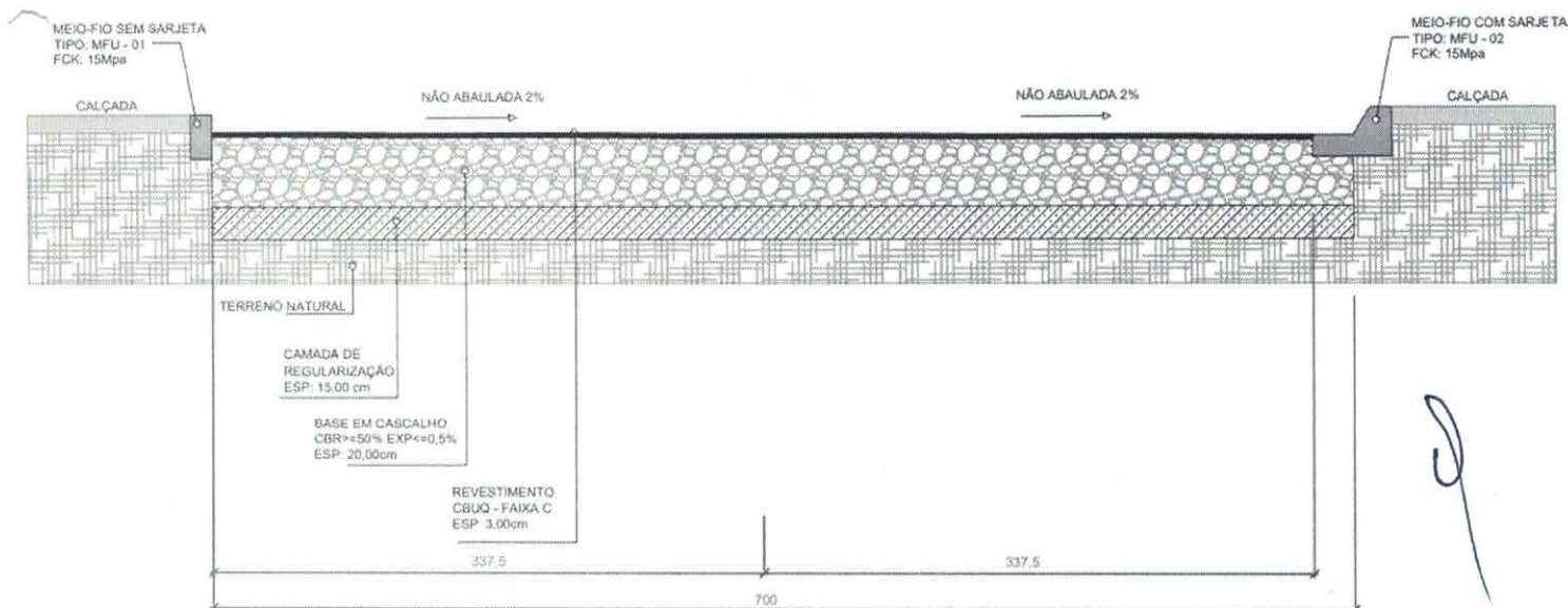
Figura 01 – Seção Transversal
