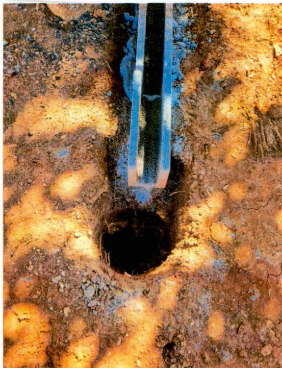
Foto 03: Furação de estaca do muro
