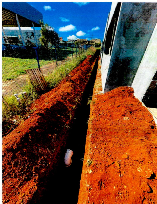
Foto 3: Drenagem de águas pluviais.
