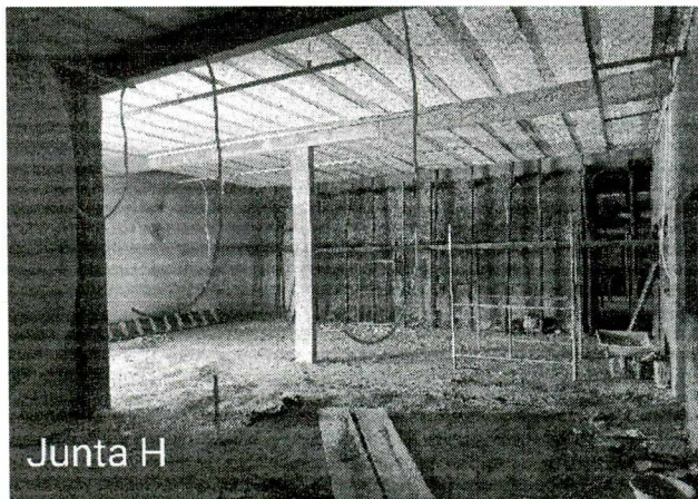
Fotos 21 a 24: Regularização de contrapiso; execução de reboco da platibanda; execução de alvenaria e regularização da calha; execução de instalações pluviais (cobertura);
