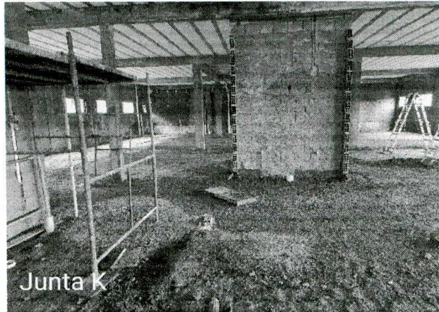
Fotos 34 a 36: Execução de alvenaria da platibanda e da calha; execução de reboco da platibanda; execução de chapisco interno e externo; execução de instalações hidrossanitárias;
