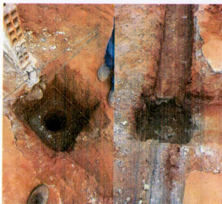
Foto 04: Escavação de valas para estacas, blocos e vigas baldrames
