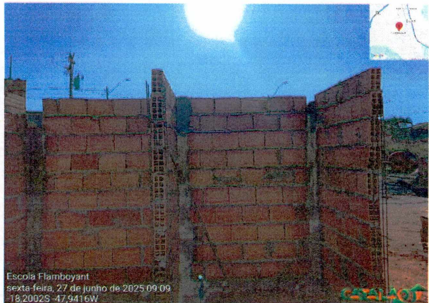
Fotos 06 e 07: Levantamento da alvenaria da central de gás e instalação do reservatório.
