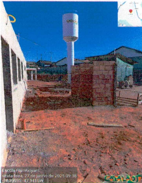
Fotos 06 e 07: Levantamento da alvenaria da central de gás e instalação do reservatório.
