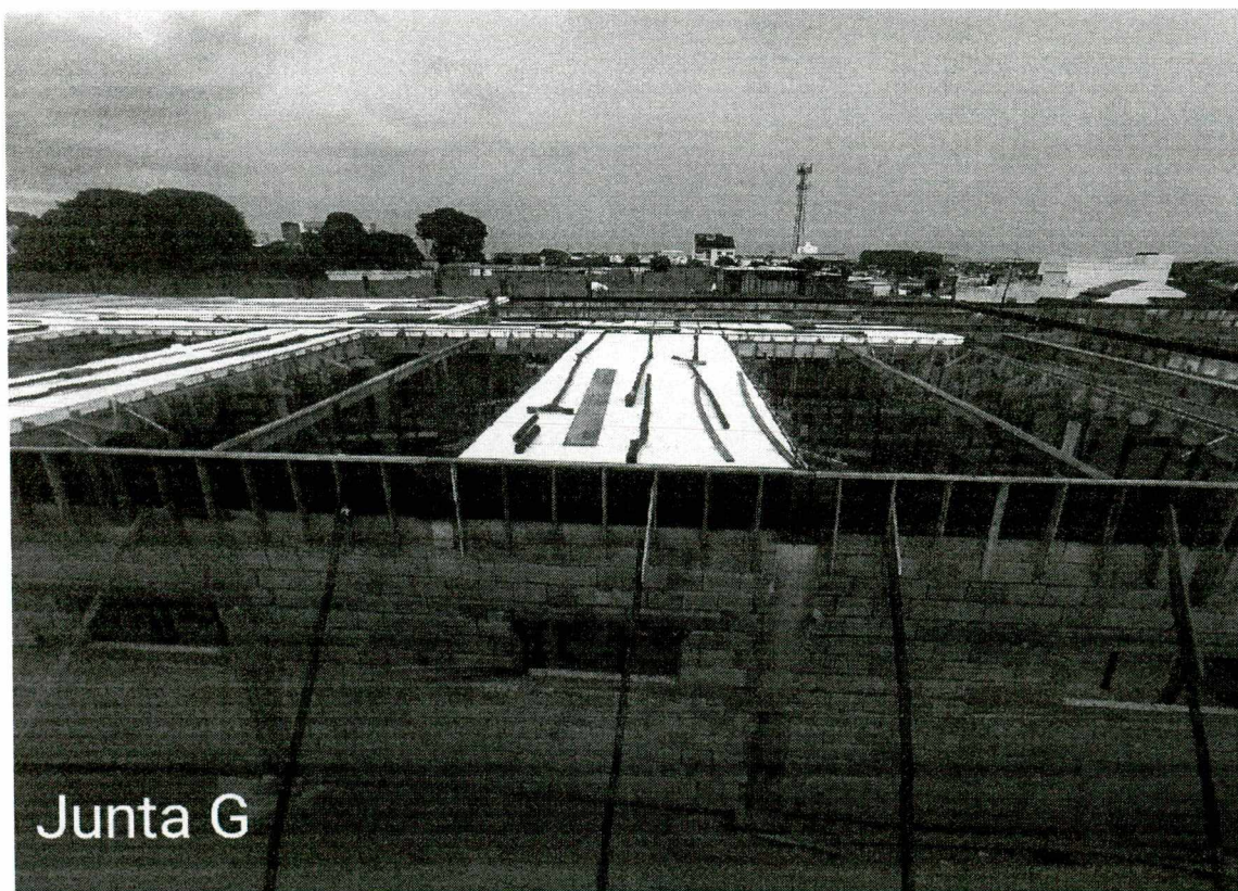
Foto 14 – Montagem das vigas de cobertura, montagem do escoramento e montagem da laje protendida
