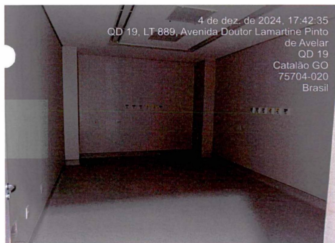
Fotos 10 a 13: Execução de piso vinílico, execução de pintura, instalação de tanques de escovação; instalação de luminárias.
