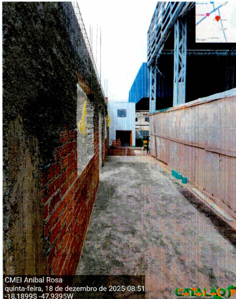
Fotos 05, 06, 07, 08 e 09: Chapisco das salas novas executado parcialmente.
