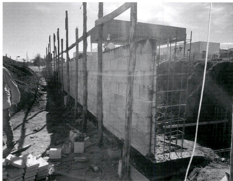
Foto 5: Construção muro de arrimo
