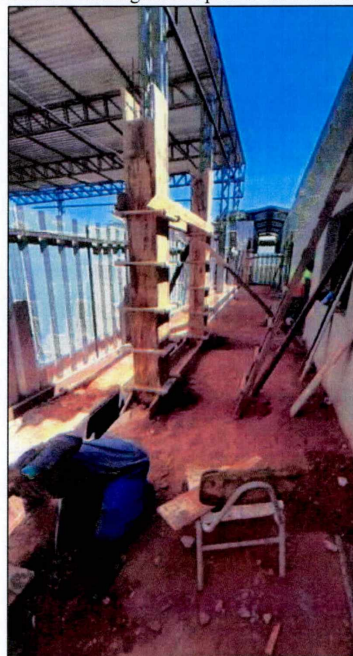
Foto 02: Execução de fôrmas e concretagem dos pilares da estrutura do telhado (Corredor 02)
