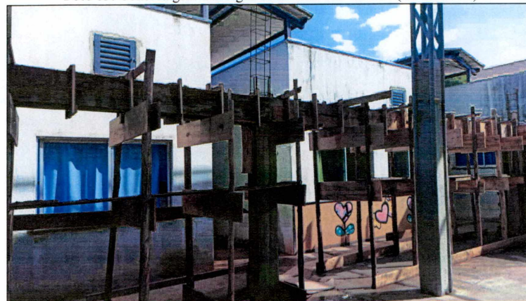
Foto 03: Concretagem das vigas da estrutura do telhado (Corredor 03)
