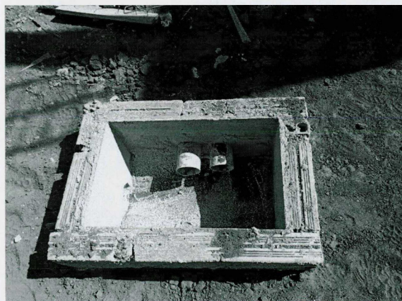
Foto 5: Execução das caixas de passagem da água pluvial
