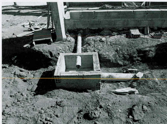
Foto 4: Execução da tubulação da água pluvial (condutor horizontal)
