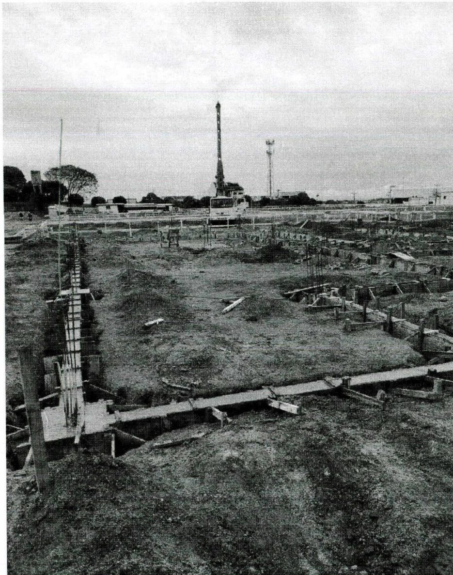
FOTO 7 – JUNTA E: Concretagem de baldrame.
