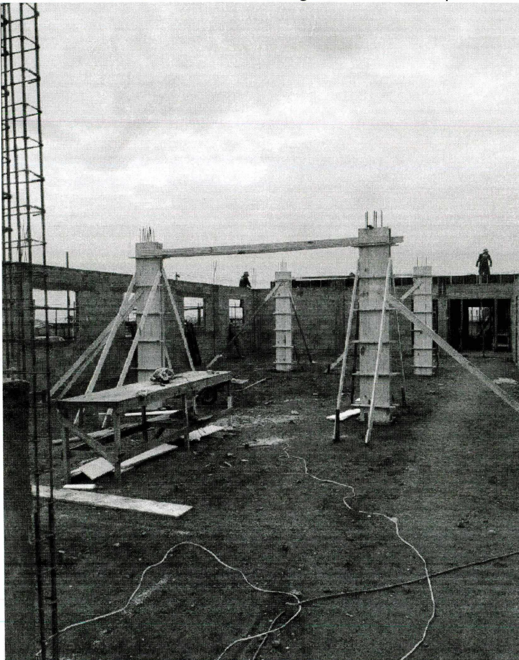
FOTOS 5 – JUNTA C: Conclusão de alvenaria montagem de formas de pilares.
