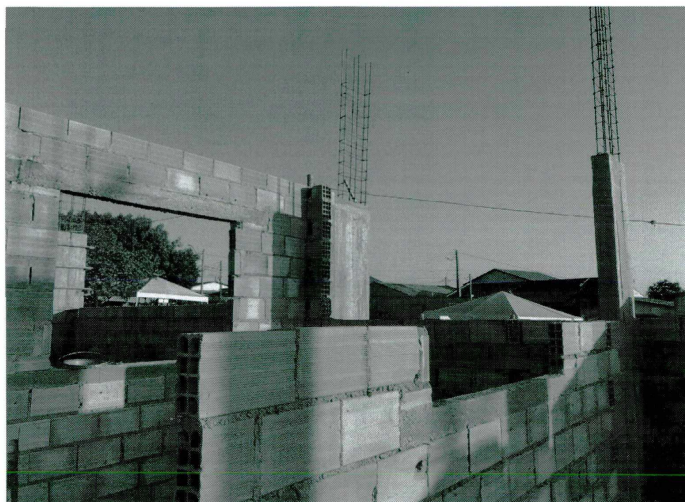
Foto 6: Concretagem de pilares da superestrutura; execução de vergas e contra-vergas.
