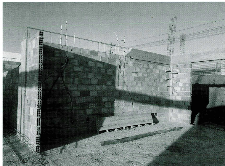
Foto 1: Execução de alvenaria e instalação de eletrodutos.
