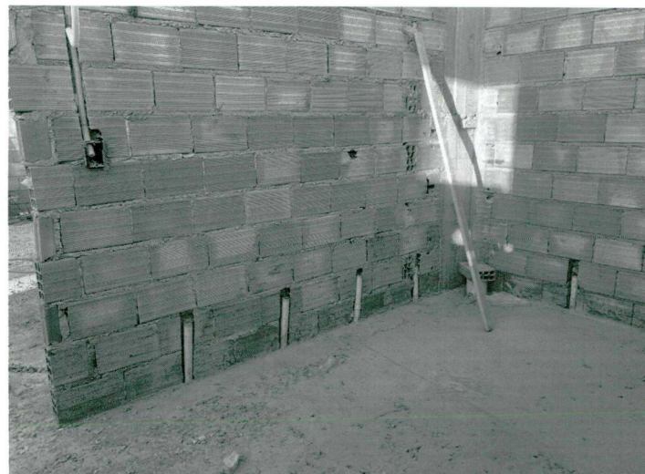
Foto 2: Execução de contrapiso, instalação de esgoto.
