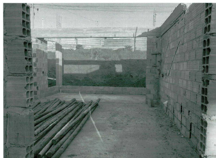
Foto 5: Execução de contrapiso, e vigas da superestrutura.
