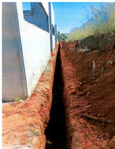
Foto 1: Escavação de vala da tubulação de esgoto
