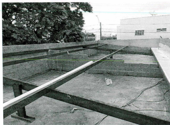
Foto 03: Execução da estrutura metálica do telhado
