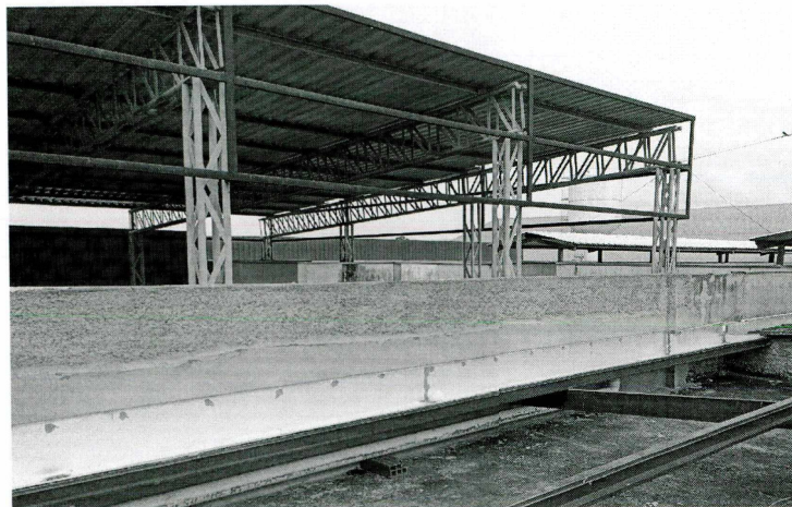
Foto 02: Execução de calhas no telhado
