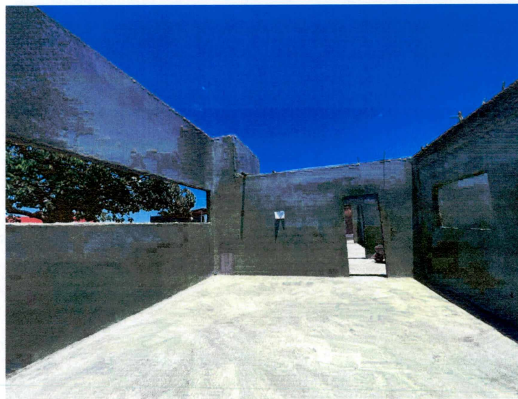
Foto 1: Reboco e contrapiso.
