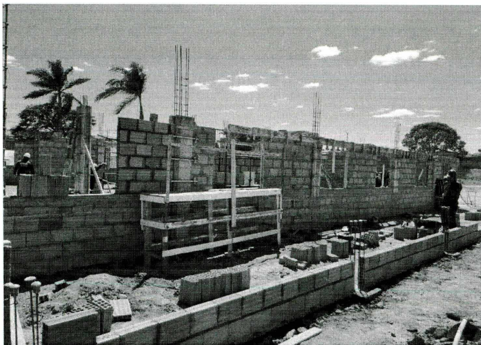
FOTOS 1 E 2 – JUNTA A: Pilares finalizados, montagem de vigas aéreas e alvenaria restante
