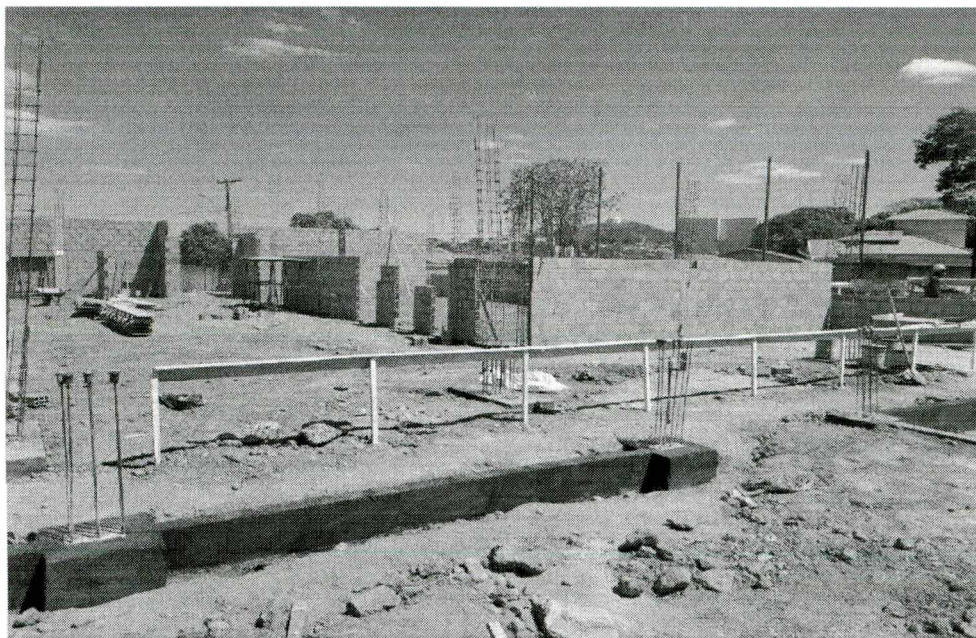
FOTOS 3 E 4 – JUNTA B: Levantamento de alvenaria, armação e montagem de forma de pilares
