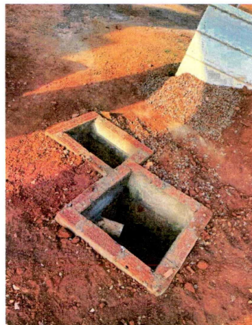
Foto 2: Drenagem de águas pluviais.
