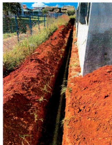
Foto 3: Drenagem de águas pluviais.
