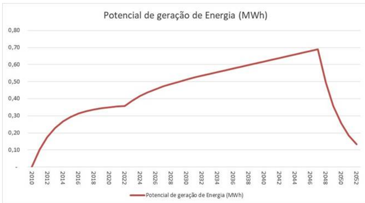
Figura 5 - Produção Estimada de Energia
