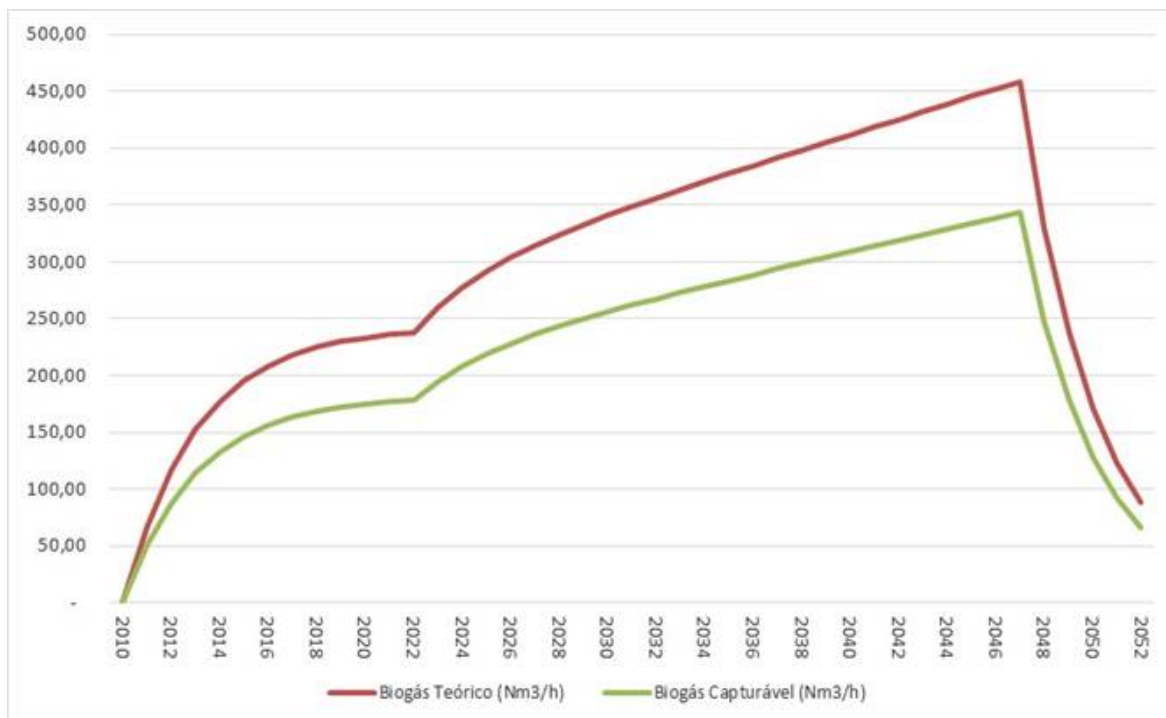
Figura 4 - Curva de Produção de Enriquecimento de Biogás
