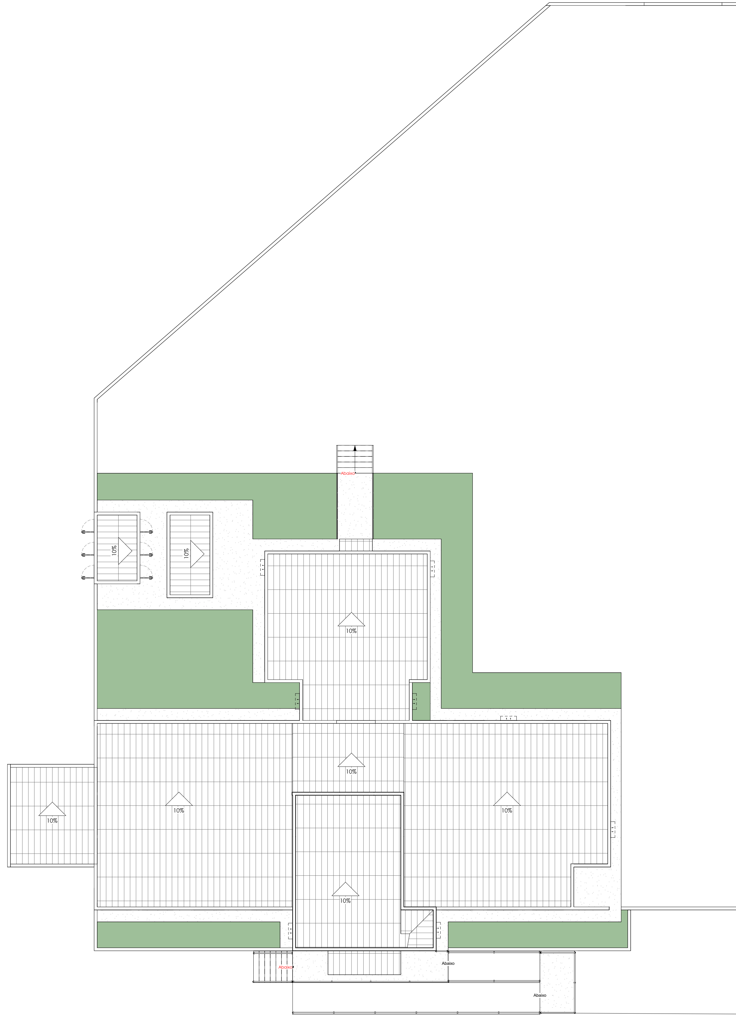
Planta de Cobertura Esc.: 1:100
