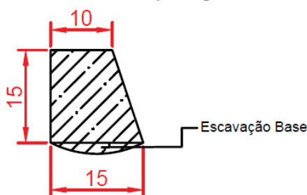
Figura 3 – Meio fio sem Sarjeta tipo MFU01.
