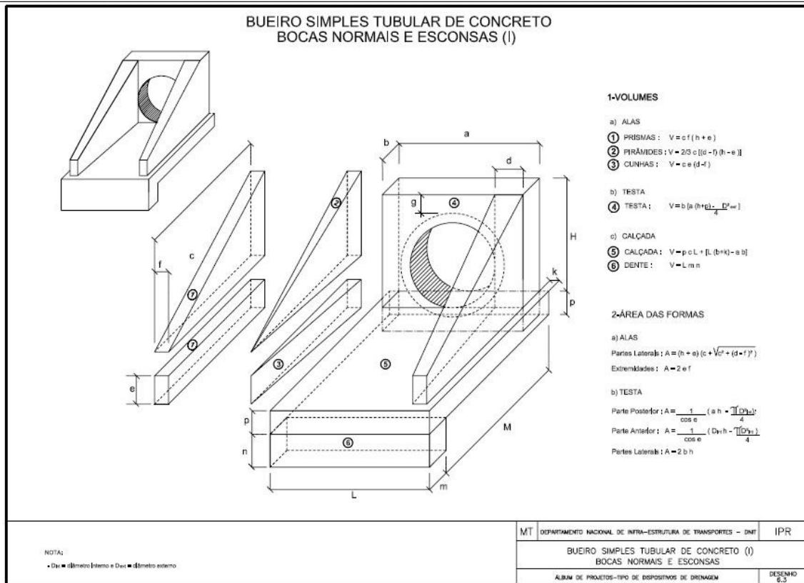
Figura 8: Dimensões - Bueiro Simples Tubular de Concreto
